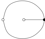
Fig. 3. The dessin d'enfant \Gamma_1 associated to H
